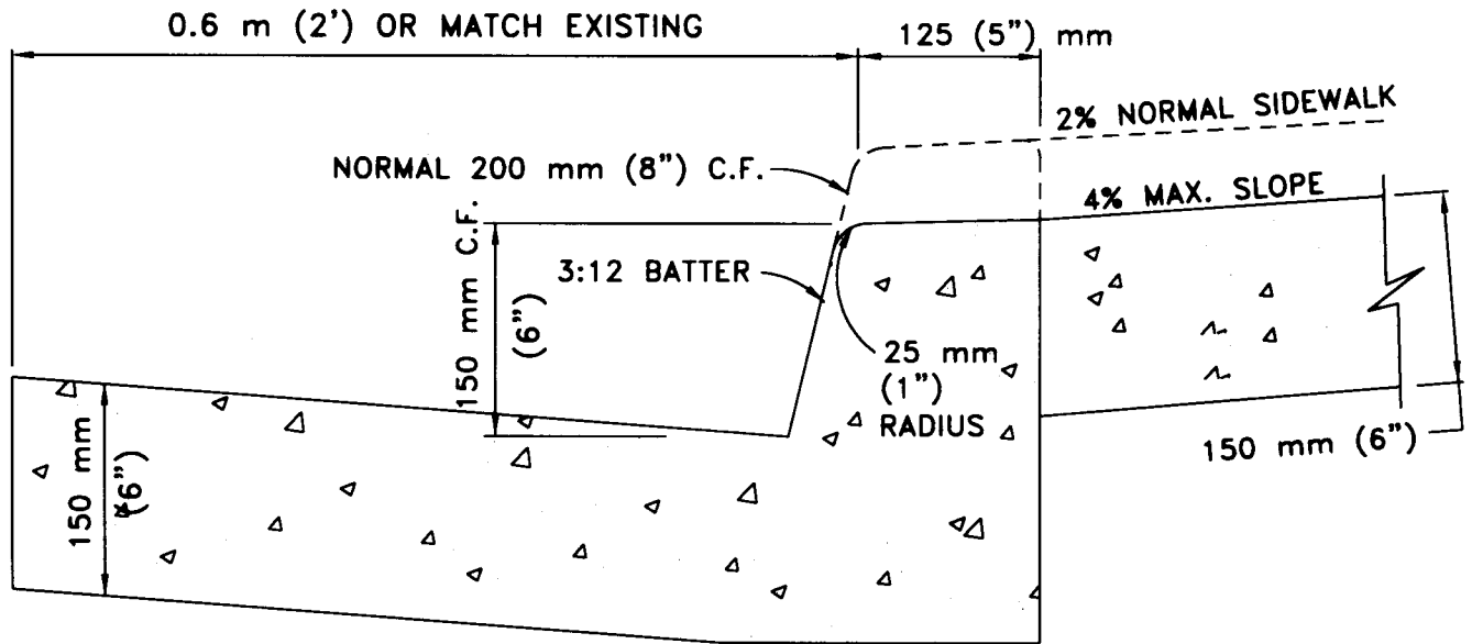
SECTION A-A SCALE: 1:6
